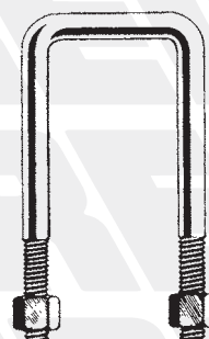
5 - 722060 \varnothing 20x90x145 6 - 722061 \varnothing 20x90x160 7 - 722063 \varnothing 20x90x180 8 - 722064 \varnothing 20x90x200 9 - 722065 \varnothing 20x90x220 10 - 722067 \varnothing 20x90x230 11 - 722066 \varnothing 20x90x240
