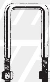
9 - 722510 \phi 14x70x130 10 - 722511 \phi 14x70x140 11 - 722512 \phi 14x70x150
