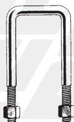
16 - 722061 ø 20x90x160 17 - 722063 ø 20x90x180 18 - 722064 ø 20x90x200 19 - 722065 ø 20x90x220 20 - 722067 ø 20x90x230 21 - 722066 ø 20x90x240 22 - 722068 ø 20x90x260
