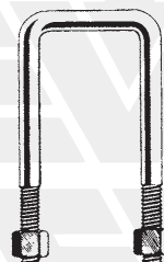
8 - 722063 \varnothing 20x90x180 9 - 722064 \varnothing 20x90x200 10 - 722065 \varnothing 20x90x220
