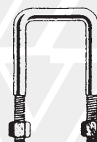
6 - 722733 \varnothing 14x80x80 7 - 722219 \varnothing 14x80x100
