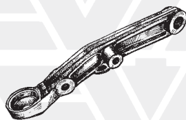
8 - 727415 Sx / LH NEW 9 - 727416 Dx / RH NEW
